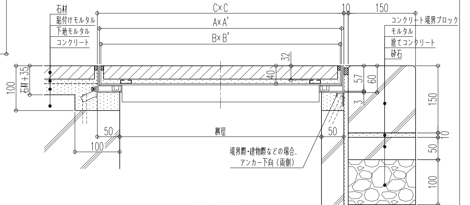
施工参考図
